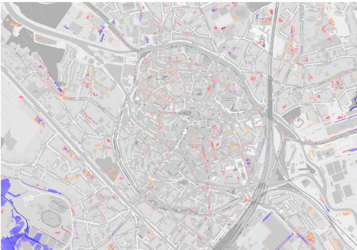
Figuur 5: Waterdiepte bij overstrooming in het huidig klimaat voor een T25-composietbui zoals opgenomen in de VLAGG-kaart. Ook historische meldingen van wateroverlast zijn aangeduid (bron: (Sweco, 2019).
