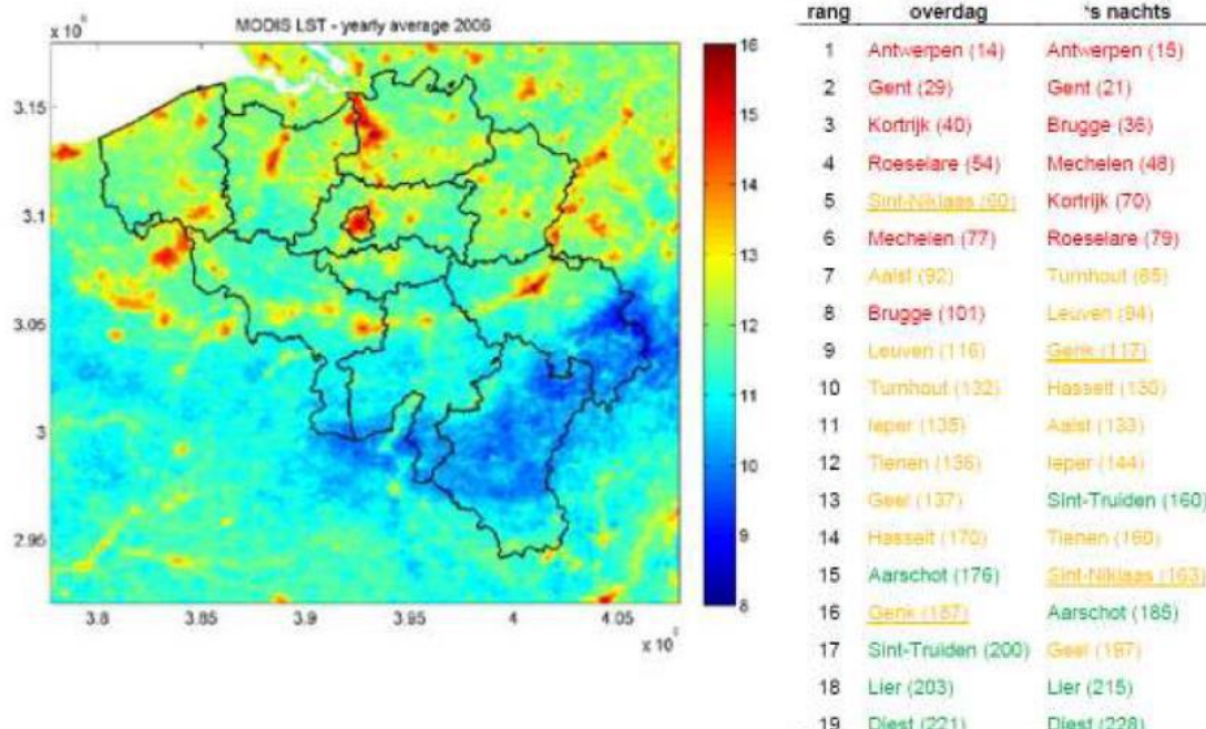
Figuur 76: Afbelding van de jaargemiddelde oppervlaktetemperatuur voor België 2006 en rangschikking volgens de sterkte van het hitte-eilandeffect op basis van oppervlaktetemperaturen (SUHI) in de zomer (april-september) over de jaren 2002-2013.
