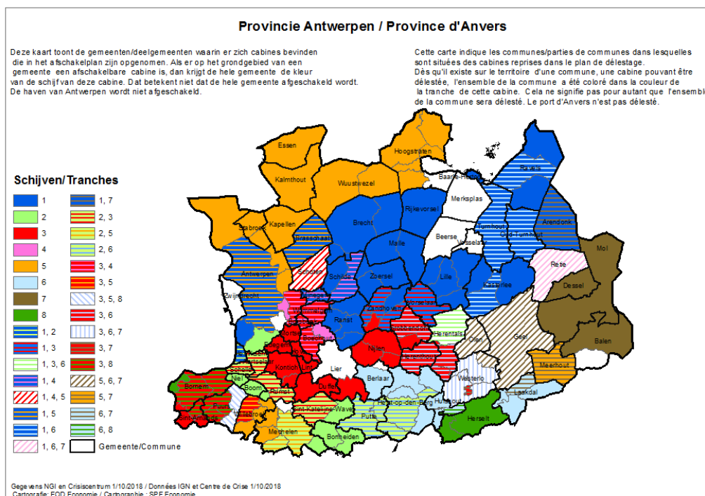
Figuur 72: Afschakelplan provincie Antwerpen (Bron: (Fluvius))
